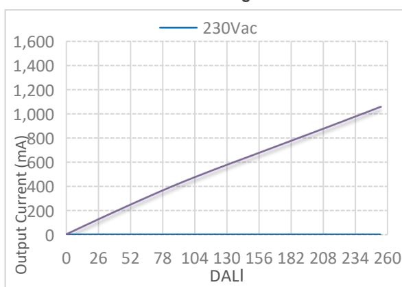
Linear dimming
